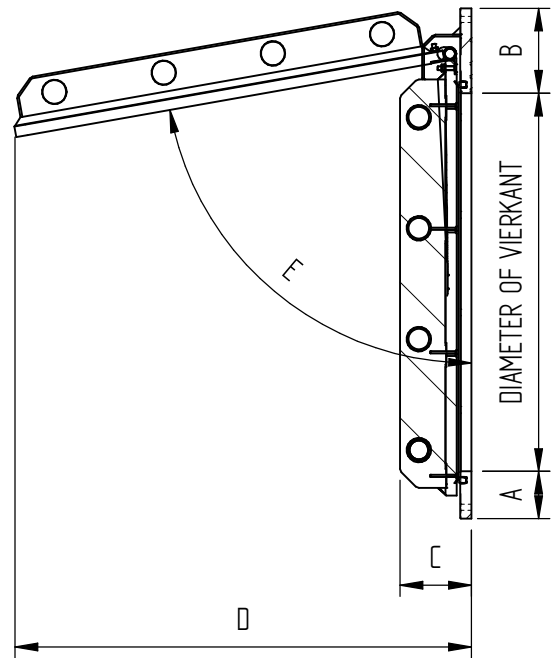
DOORSNEDE A-A
